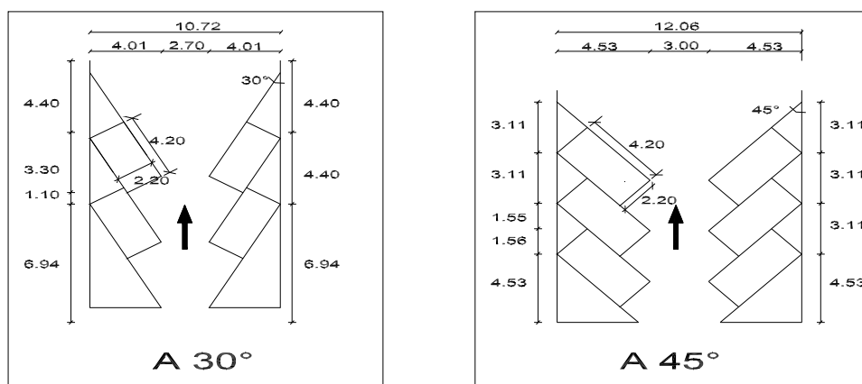
DIBUJO 1.2.2-D. AUTOS CHICOS
