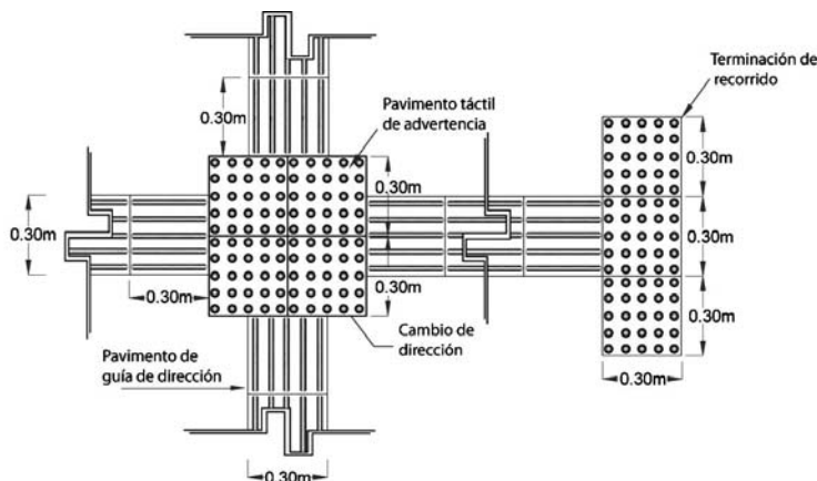
DIBUJO 2.3.7-D. CAMBIO DE DIRECCION CUATRO MÓDULOS – PLANTA
