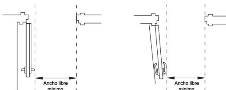
DIBUJO 4.1.1-A. PUERTA ANCHO LIBRE - PLANTA
